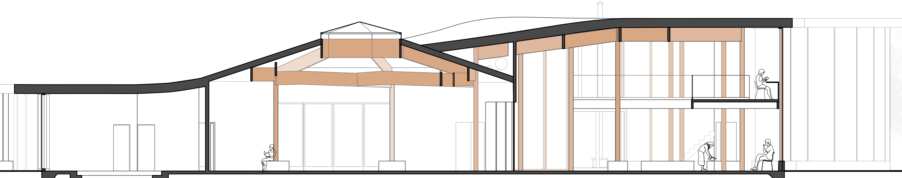
COUPE A 1:100
